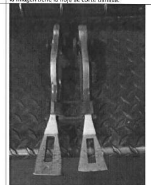
Equipos para rescate con más de 8 años de uso. El de la imagen tiene la hoja de corte dañada.
