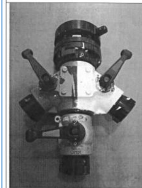
Accesorios para abastecimiento en maniobras contra incendios antiguos, sellos deficientes haciendo que se pierda agua.
